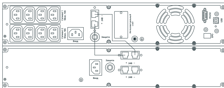
Рисунок 7. Стандартная установка ВБМ
