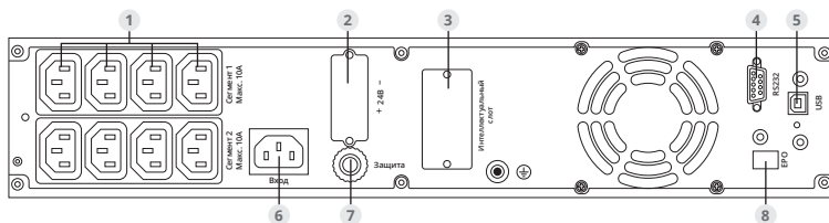
Рис. 1: Вид сзади: ИБП ИМПУЛЬС ФРИСТАЙЛ 1000-2000 ВА
